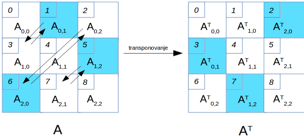
Slika 3.12: Transponovanje matrice kada je P = Q = \text{NZD} = 3 . Čvorovi transponuju sve tri \text{NZD} dijagonale u jednom koraku.
