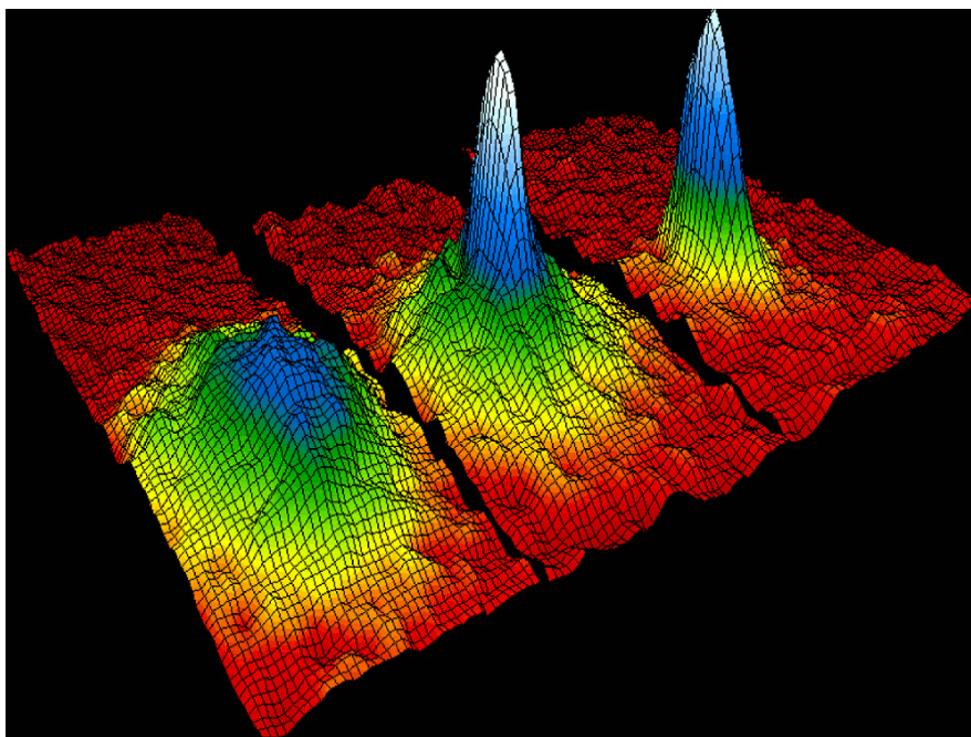
Slika 1.1: Eksperimentalni rezultati grupe Wolfganga Keterlea iz 1995. godine [5] kojima je pokazana pojava Boze-Ajnštajn kondenzacije ispod kritične temperature. (By NIST/JILA/CU-Boulder - NIST Image, Public Domain, https://commons.wikimedia.org/w/index.php?curid=403804 )
