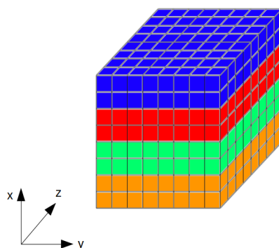
Slika 2.4: Ravnomerna distribucija podataka po X osi na računarskom klasteru. Različite boje predstavljaju skupove podataka koje su dodeljene različitim čvorovima (u ovom slučaju 4 čvora).
