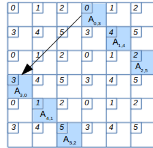
(b) treća dijagonala, A(i, i) gde je \text{MOD}(j-i, \text{NZS})=3
