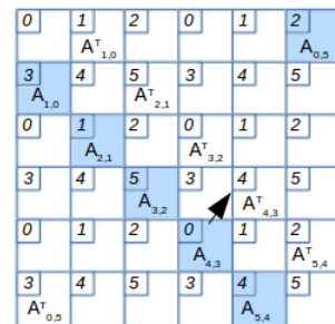
(f) druga dijagonala, A(i, i) gde je \text{MOD}(j-i, \text{NZS})=5
