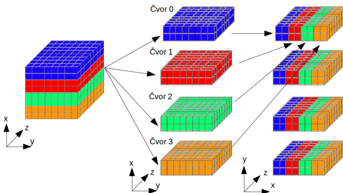
Slika 2.5: 3D transponovanje distribuiranih podataka između čvorova klastera opisano u tekstu.
